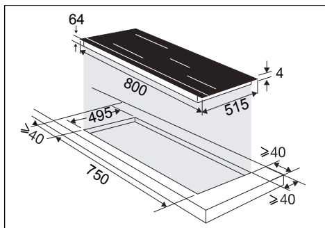
Asennus työtason päälle
