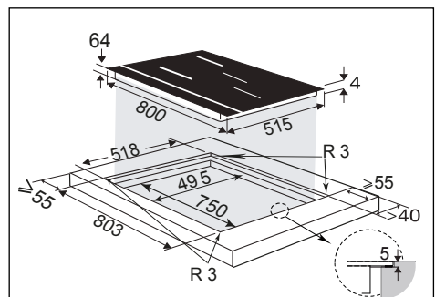
Bündiger Einbau
