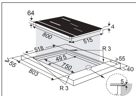
Asennus pinnan tasolle
