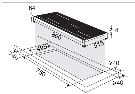
Einbau in eine Arbeitsplatte
